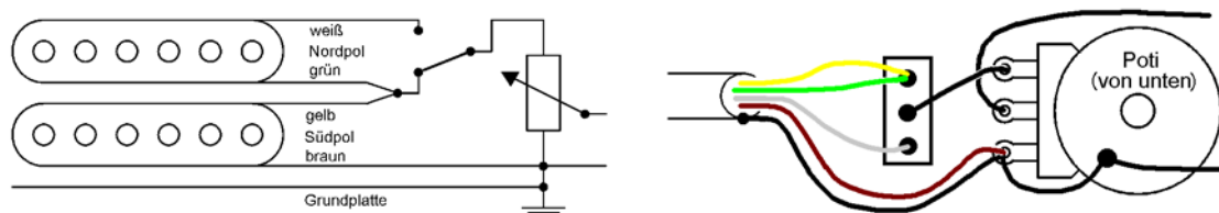
Umschaltung Humbucker / Südpolspule allein
